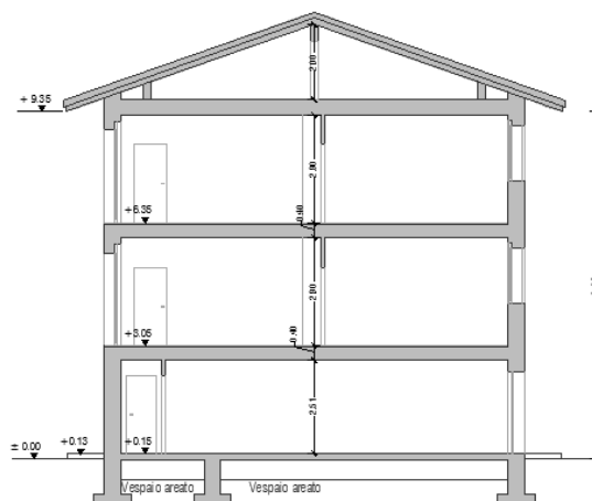
sezione C-C'
