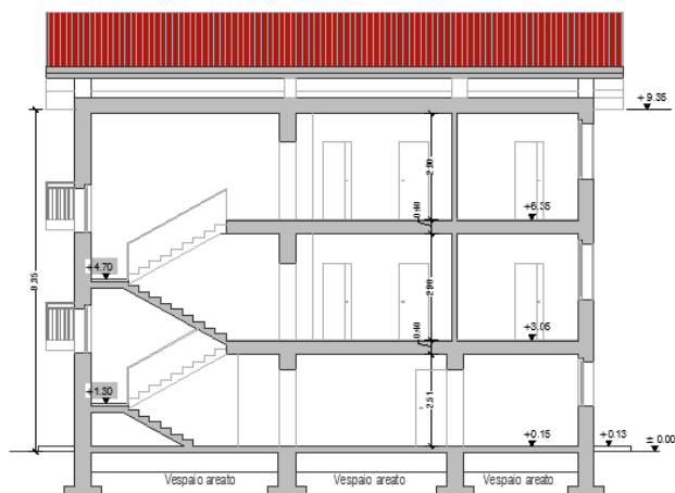
sezione B-B'
